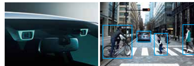
ステレオカメラ
