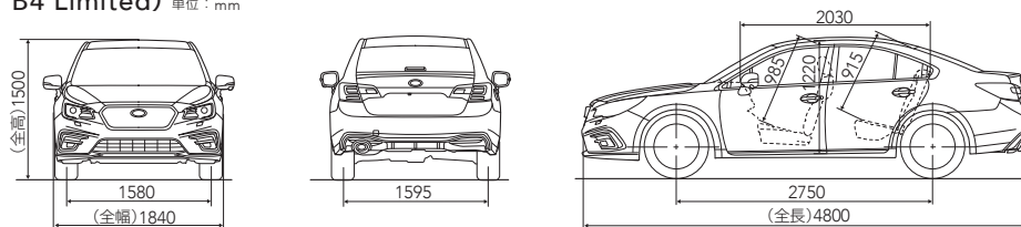
3面図(LEGACY B4 Limited) 単位: mm
