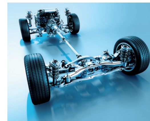
低重心・左右対称レイアウトのシンメトリカルAWD
