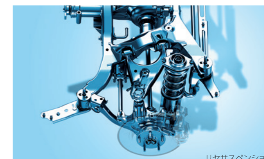
リヤサスペンション
