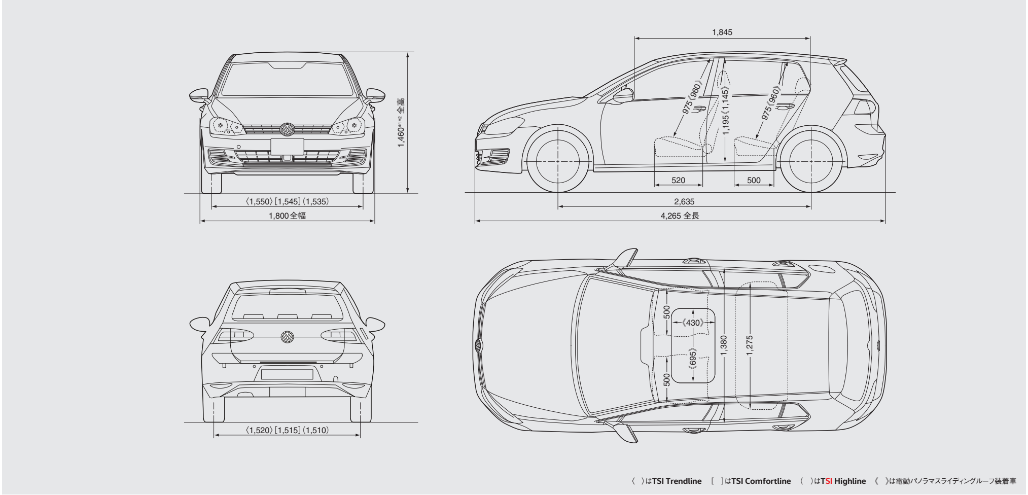
四面図(mm)
